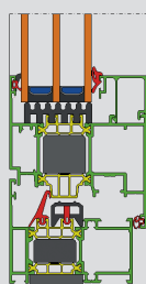
beslaggroef 16 mm (alleen design uitvoering)
